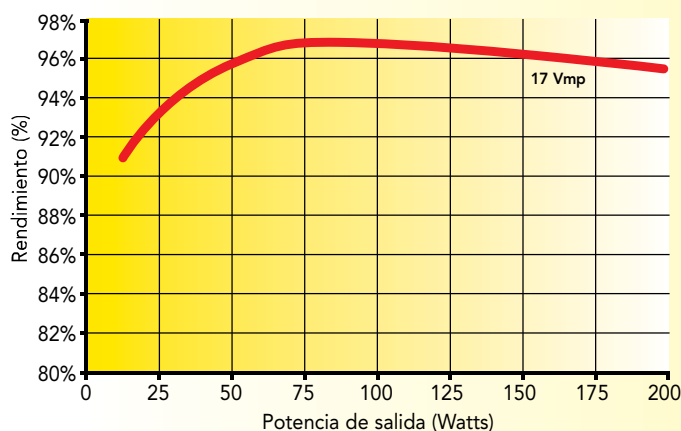
Rendimiento del SS-MPPT (12 Voltios)
